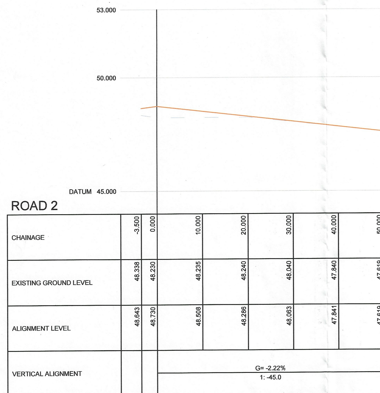
ROAD 2 - LONGSECTION SCALE: H 1:500,V 1:100. DATUM: 45.000
